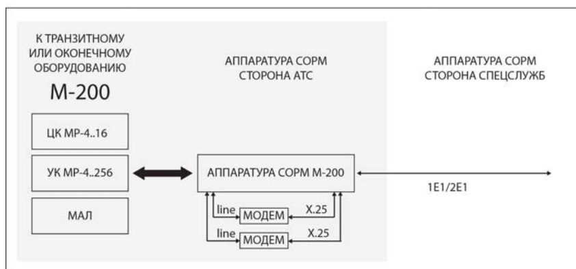
Аналоговое подключение СОРМ (приказ №70)
