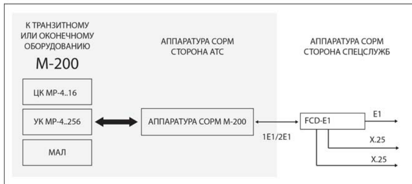
Цифровое подключение СОРМ (приказ №268/70)
