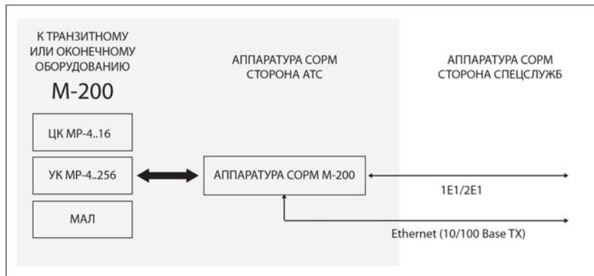
Цифровое подключение СОРМ (приказ №268)
